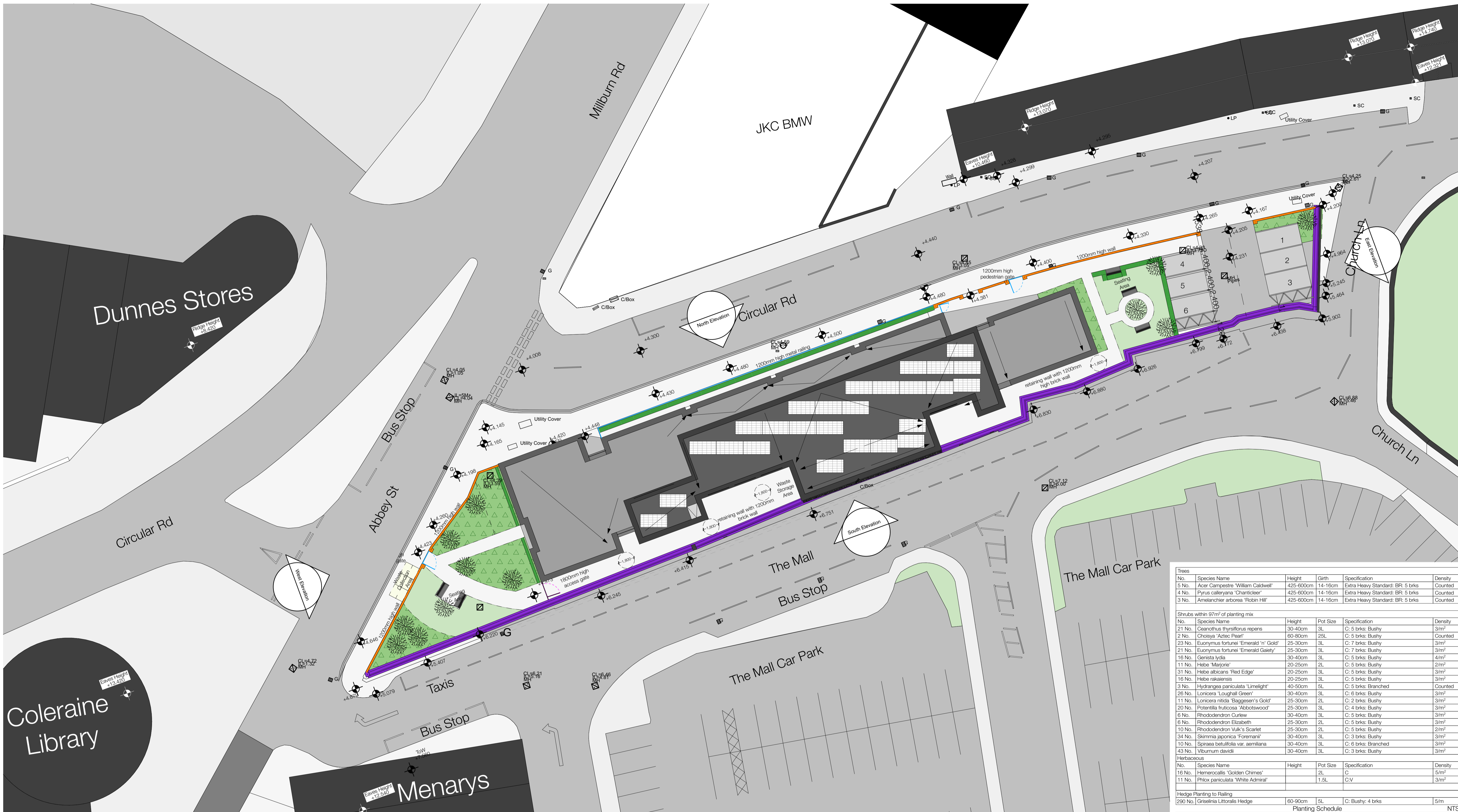
Site Plan 1:200
